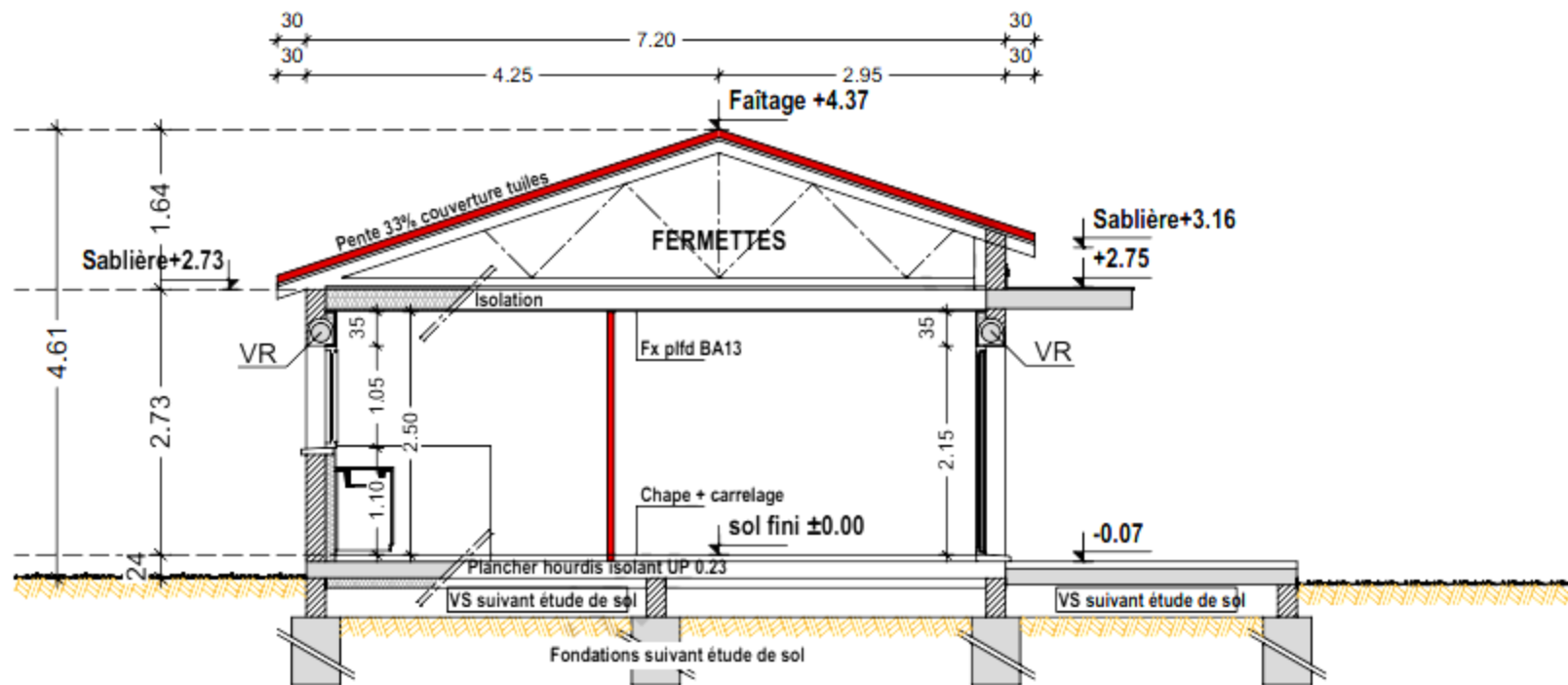
Coupe A-A
