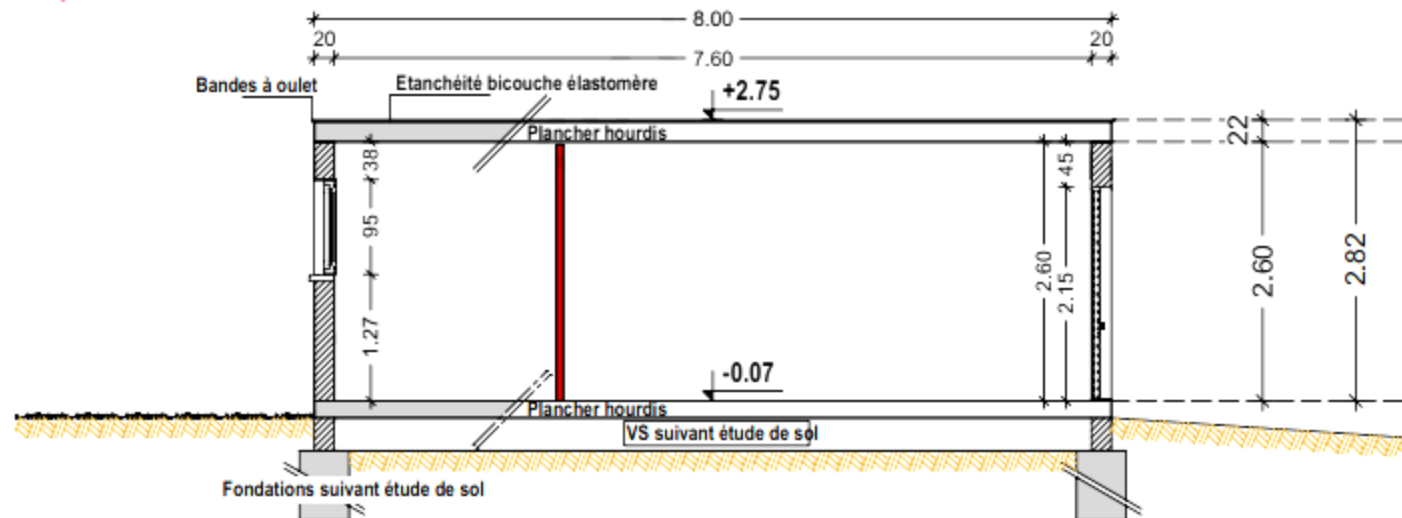
Coupe B-B
